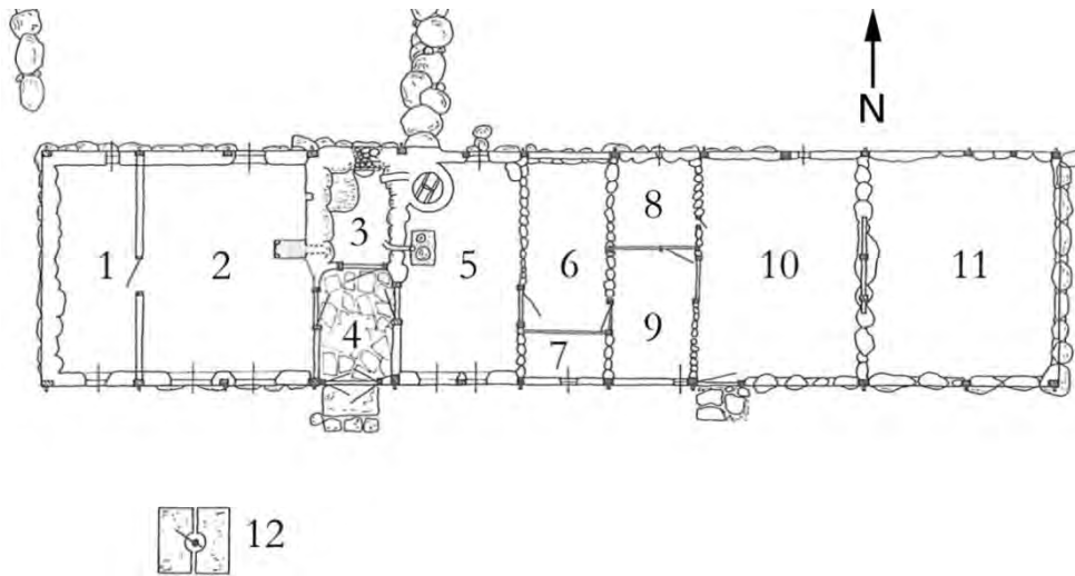
Plan över Örumshuset: 1) bagbus/ kistekammare, 2) stuga, 3) illare, 4) förstuga, 5) kök, 6) torv- och vedbod, 7) hönsbus, 8) fårkätte, 9) svinstia, 10) loge och 11) loggolv.
