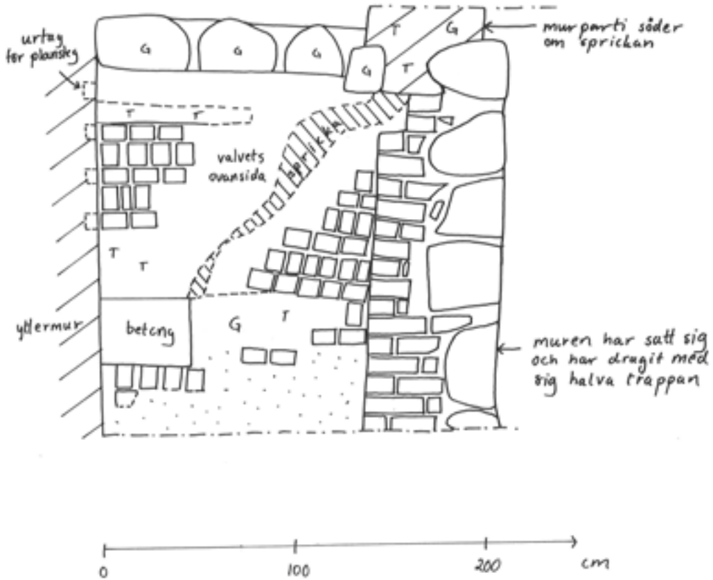
Fig. 6. Trappan sedd framifrån, 1:20. Kristina Nilén 2001-11-19.
