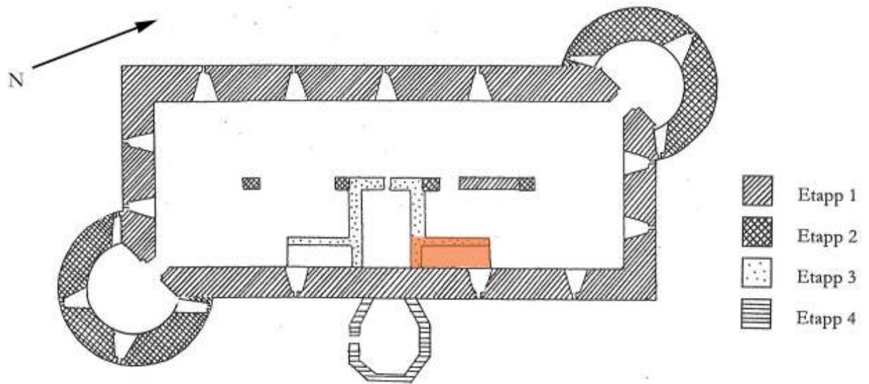
Fig. 1. Plan över Lillöbus. Norra trapparmen markerad. Notera trappans stödmurar, som bildar det lilla slutna, centrala rummet. Cecilia Pantzar 2000.
