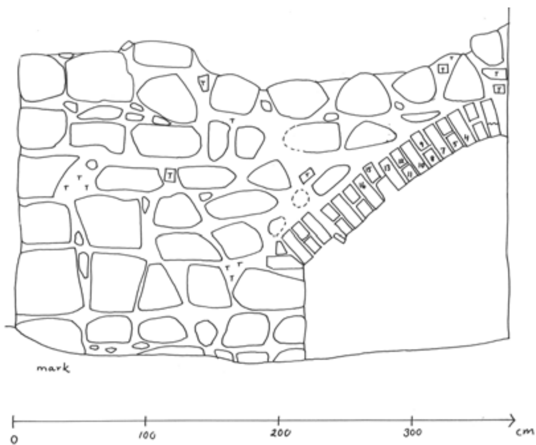
Fig. 3. Trappmur åt väster, 1:20. Kristina Nilén 2001-11-19.
