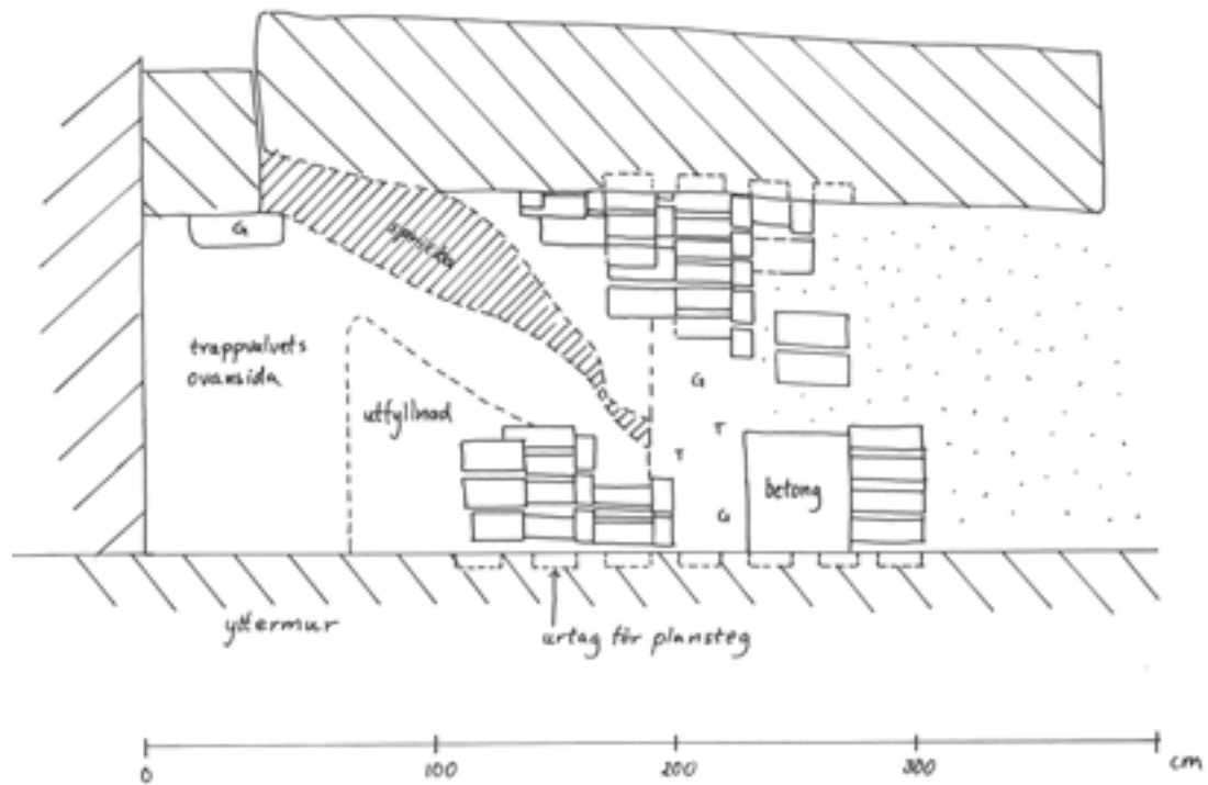
Fig. 5. Plan över trappan, 1:20. Kristina Nilén 2001-11-20.
