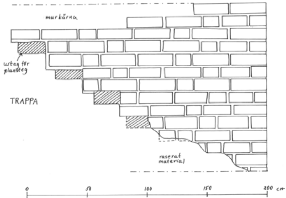
Fig. 4. Trappmur åt öster, detalj, 1:10. Kristina Nilén 2001-11-20.
