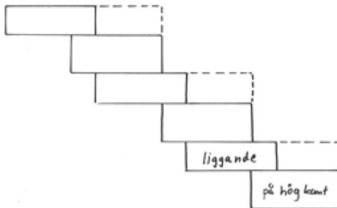
Fig. 7. Principskiss för plan- och sättsteg, genomskärning. Kristina Nilén 2001.
