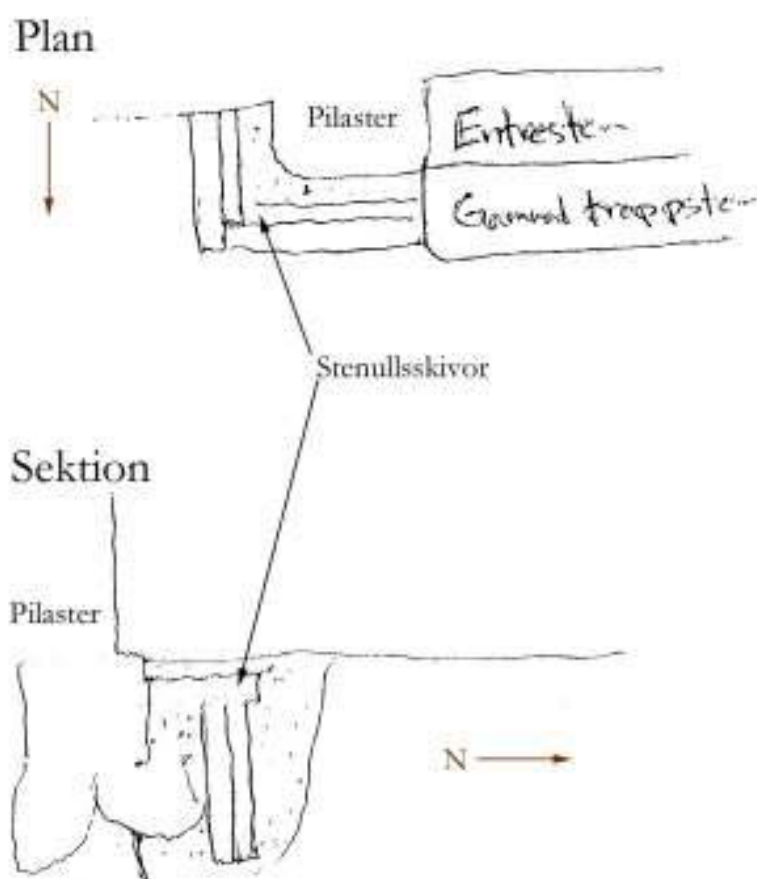
Skiss över grävning och utförd markisolering kring portalen till Nykyrkan. Utförd av Folke Carlssons byggnads AB. Skissen bearbetad av Regionmuseet i Kristianstad/Landsantikvarien i Skåne.
