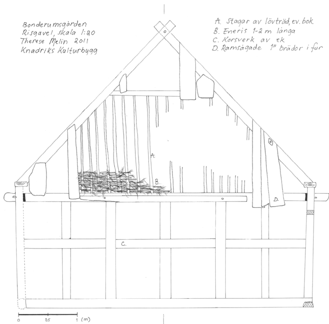
Uppmättningsritning av enrisgaveln, vy mot väster. Therese Melin, 2011.
