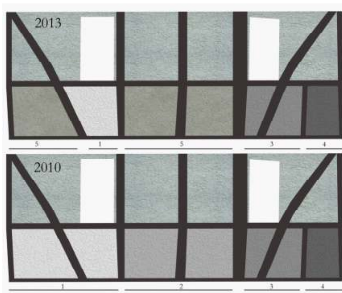
Fig. 6. Huvudbyggnadens södra gavel. Under Lerprojektet 2010 omputsades de nedre fackfyllningarna med: 1. Rent lerbruk på lersten och tegel, 2. Lerbruk med kalk (1:6) på lersten och tegel, 3. Lerbruk med kalk (1:1) på tegel och 4. Kalkbruk. Under arbetet 2013 ersattes det ena 1-materialet och bägge 2-materialen med 5; rent, fetare lerbruk på lersten och tegel. OBS, numreringen 1–5 är inte vedertagen i andra sammanhang än i denna rapport och är skapad endast i pedagogiskt syfte!
